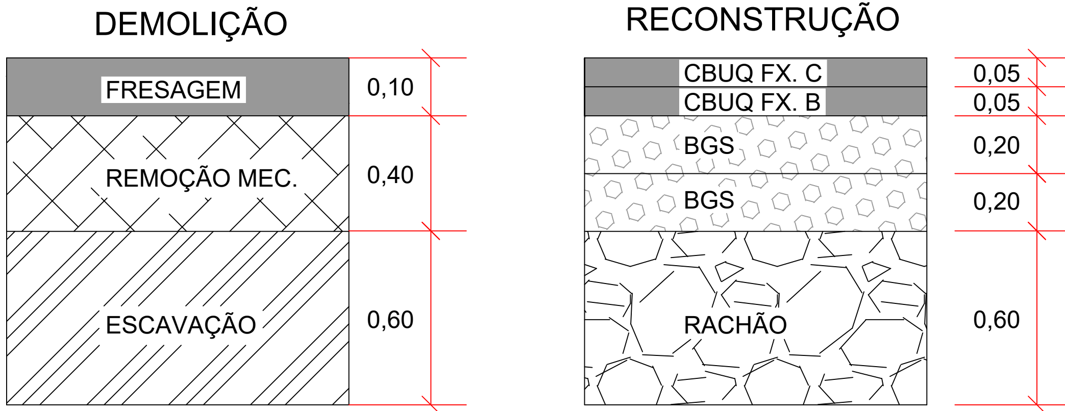
100+920 ao 100+980 (60,00 x 3,90)
