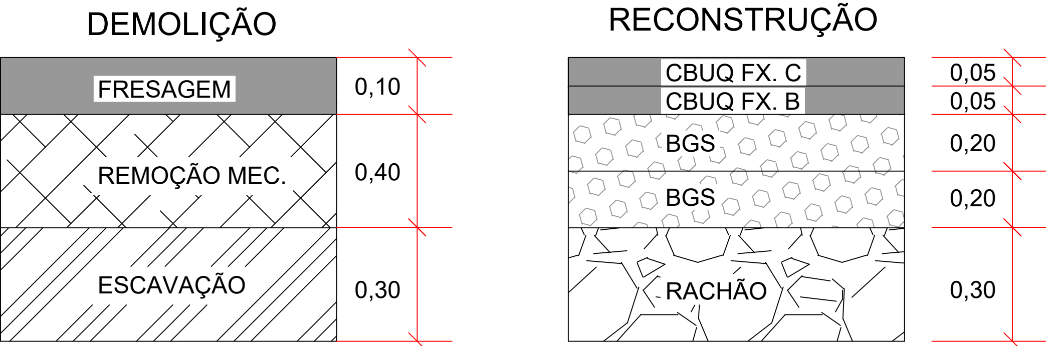
101+015 ao 101+071 (56,00 x 3,90)
