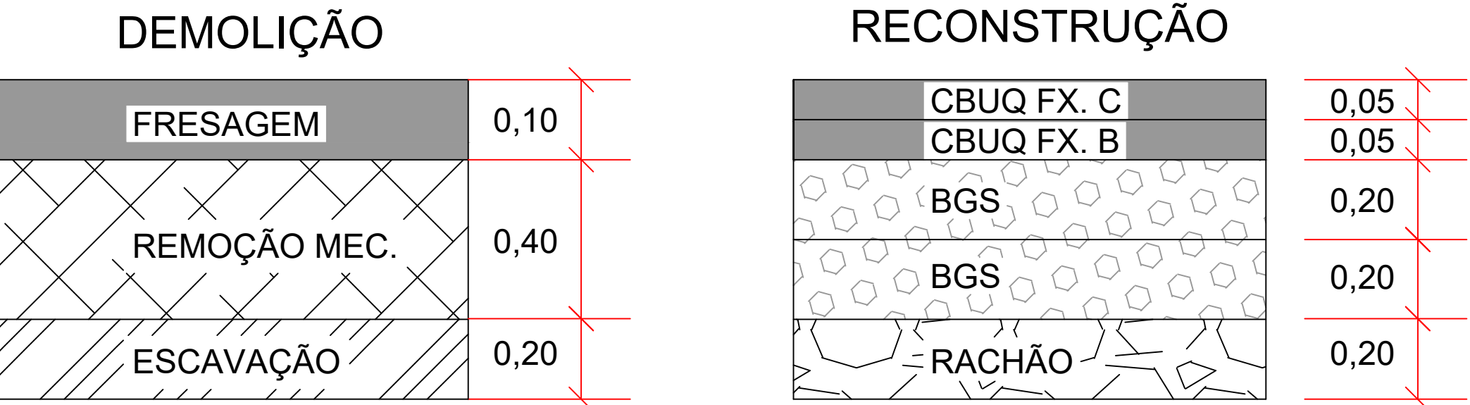
101+173 ao 101+261 (88,00 x 3,90)
